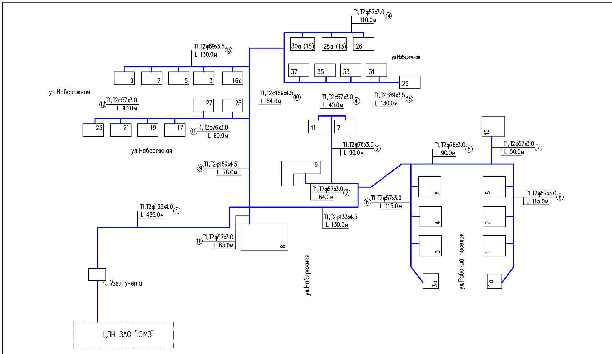
Рисунок 10. Схема тепловых секций от ТЭЦ ЗАО "ОМЗ" (микрорайон "Рабочий поселок")
