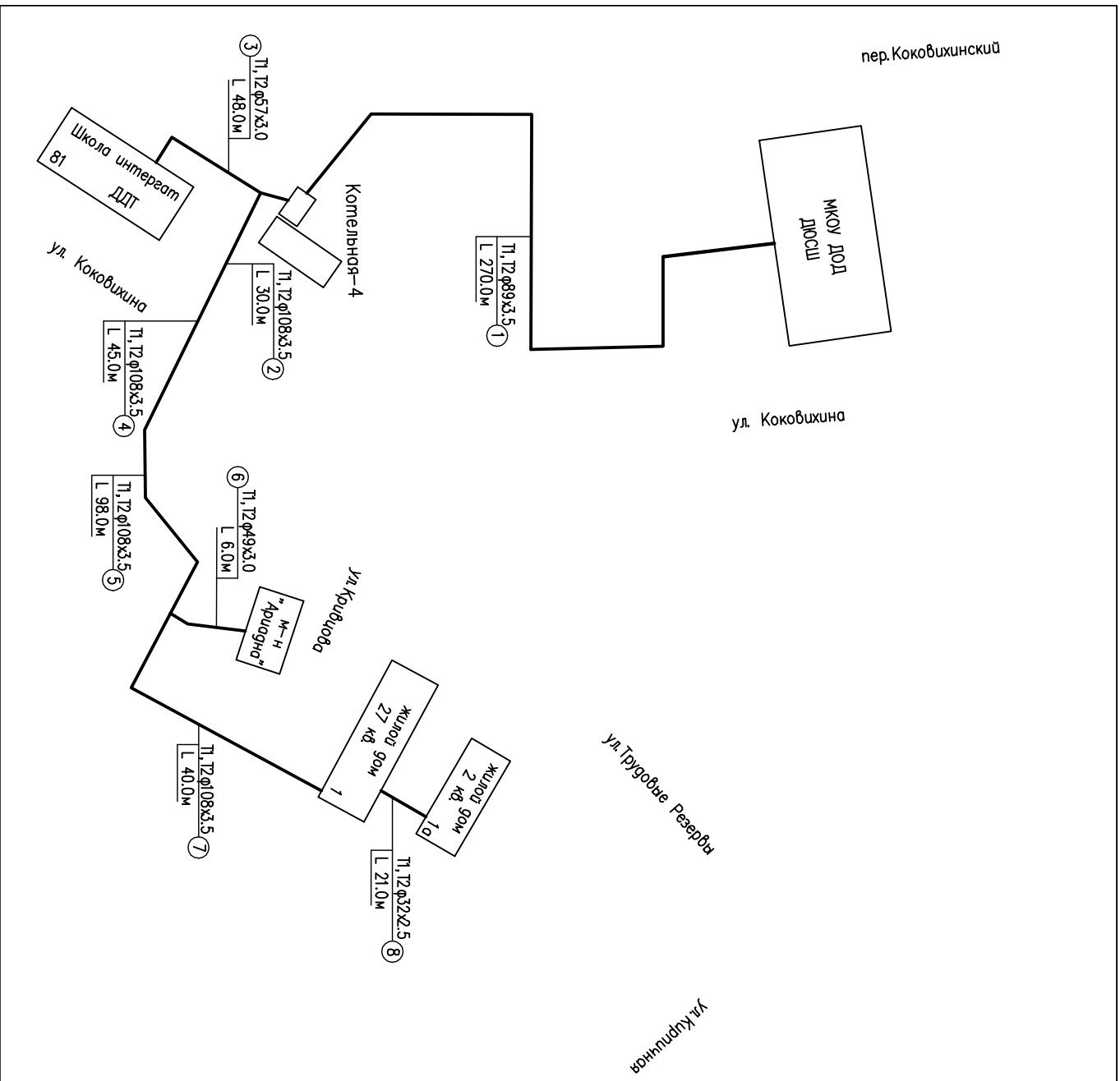
Рисунк 7. Схема тепловой секции от котельной 4 МУП ЖКХ Омутнинского района
