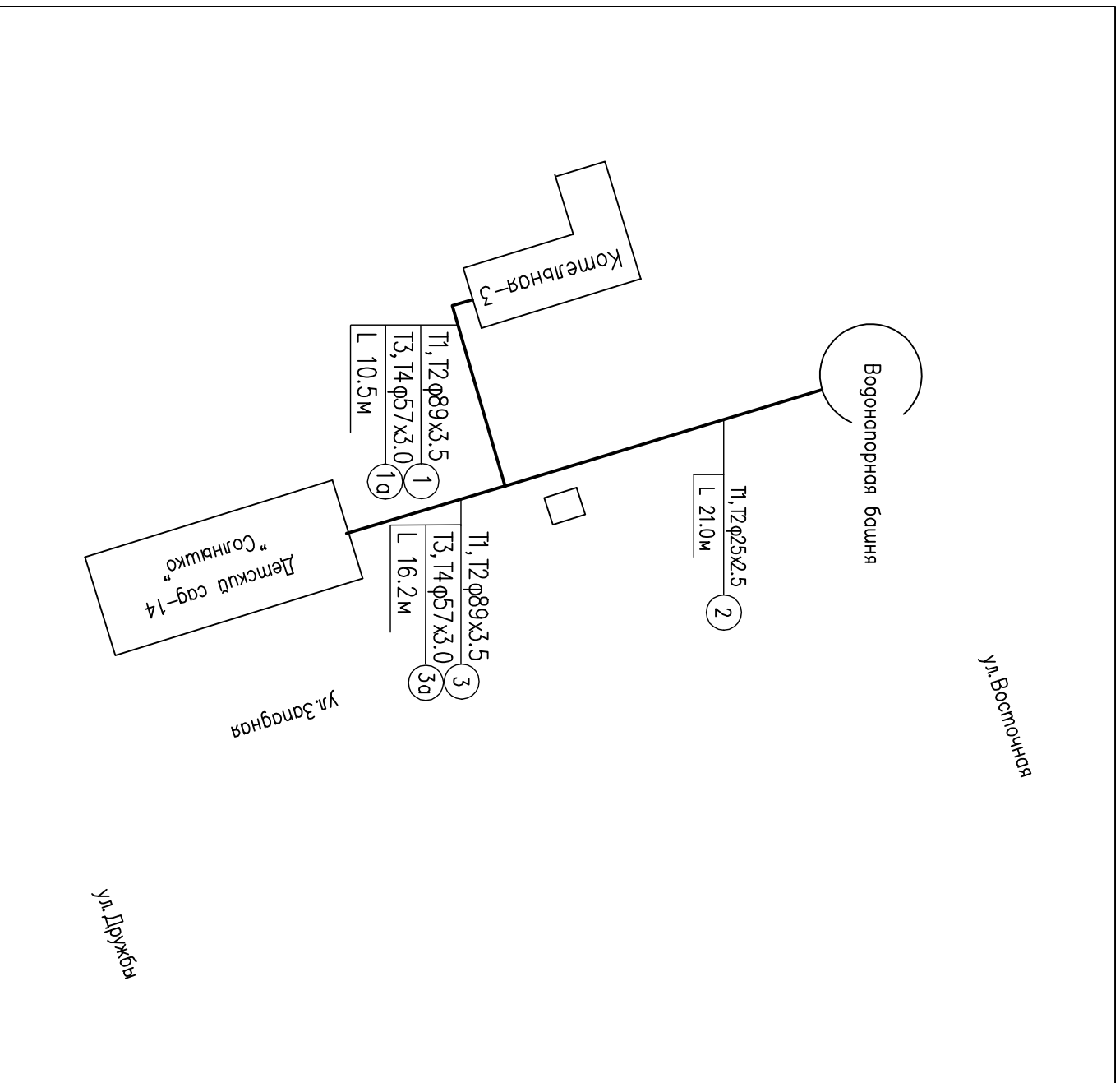
Рисунка 6. Схэма тэпловых сэктэей от котельной 3 МУП ЖКХ Омутнинского района
