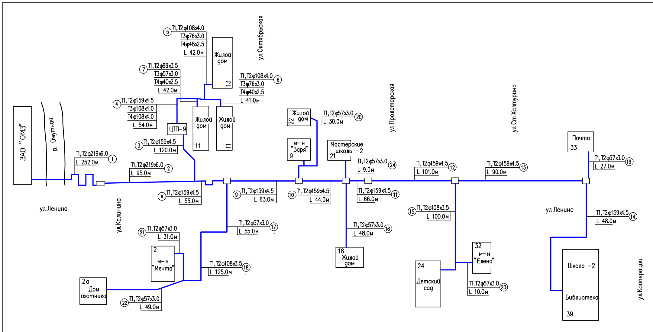
Рисунок 9. Схема тепловых секций от ТЭЦ ЗАО "ОМЗ" (микрорайон "Малагово")
