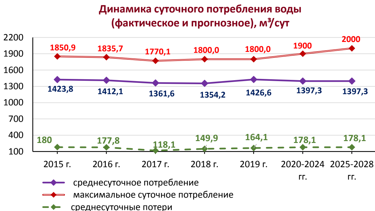
Рисунок 6. Динамика суточного потребления воды (фактическое и прогнозное)
