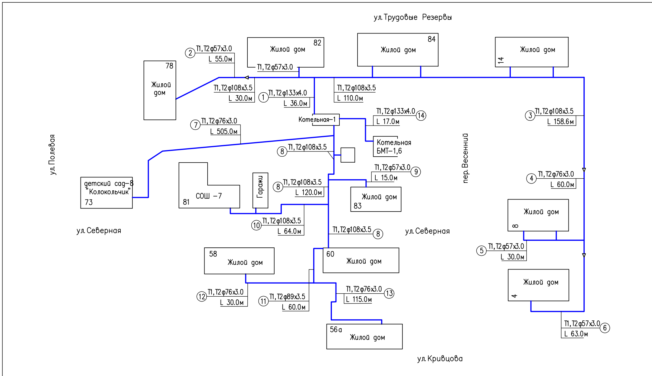
Рисунок 5. Схема тепловых секций от котельной 1 МУП ЖКХ Омутнинского района
