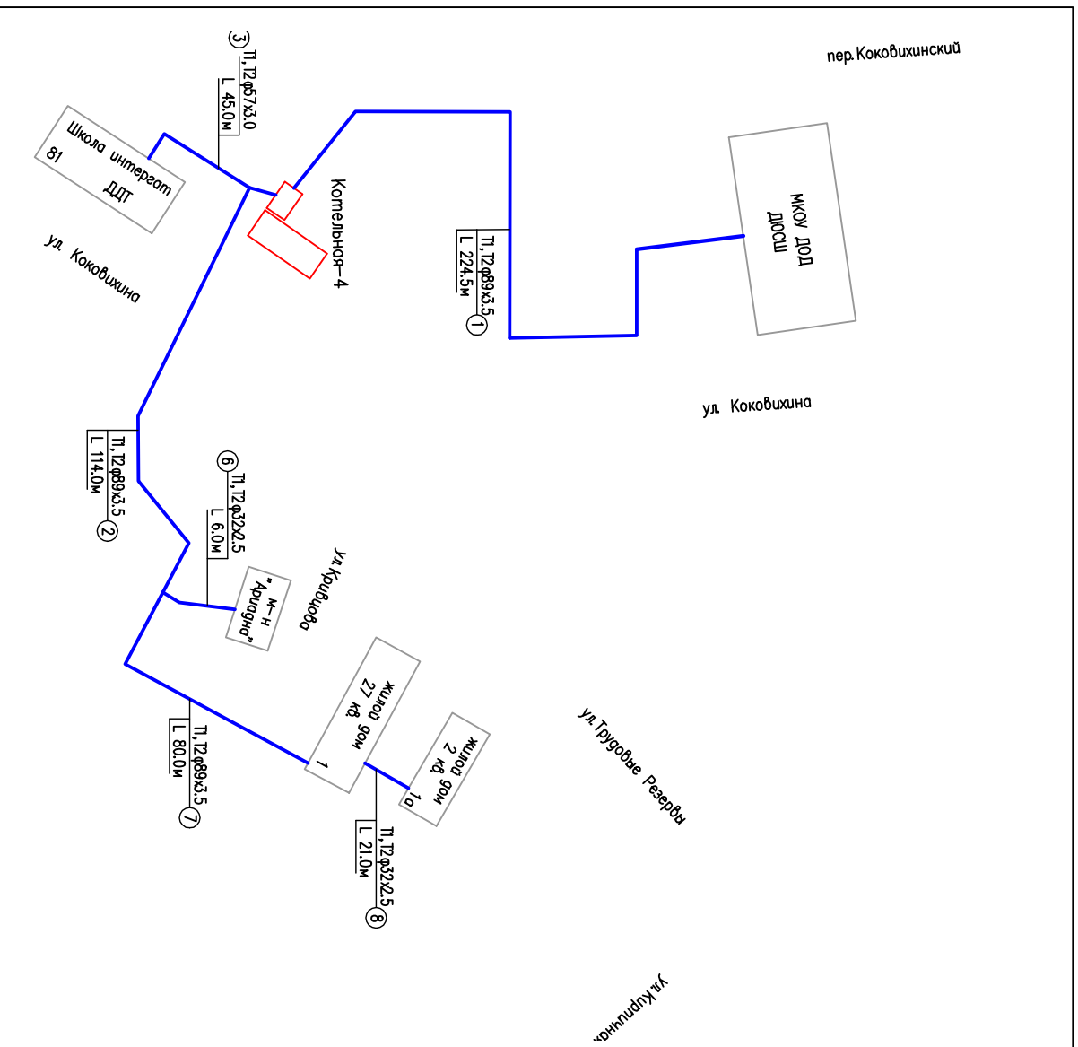
Рисунок 7. Схема тепловой сети от котельной 4 МУП ЖКХ Омутнинского района
