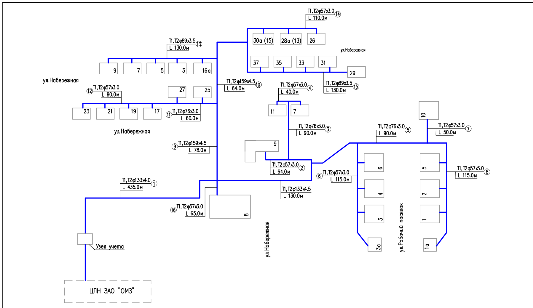
Рисунок 10. Схема тепловых сектей от ТЭЦ ЗАО "ОМЗ" (микрорайон "Рабочий поселок")
