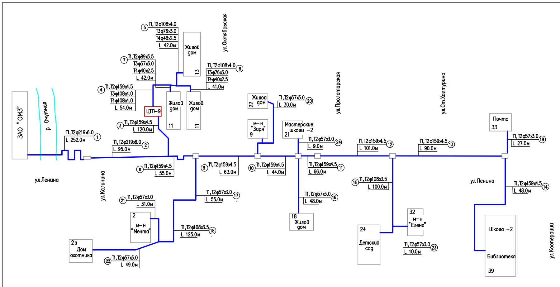
Рисунок 9. Схема тепловых секций от ТЭЦ ЗАО "ОМЗ" (микрорайон "Малагово")
