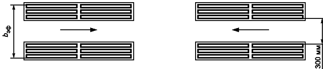
Рисунок А.6 - Форма рифления - прямолинейные параллельные риффы с плоской вершиной (6 шт.), используемые для обустройства направляющего указателя для движения в одном направлении
