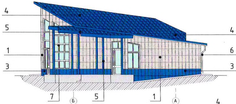
Фасад Б-А
