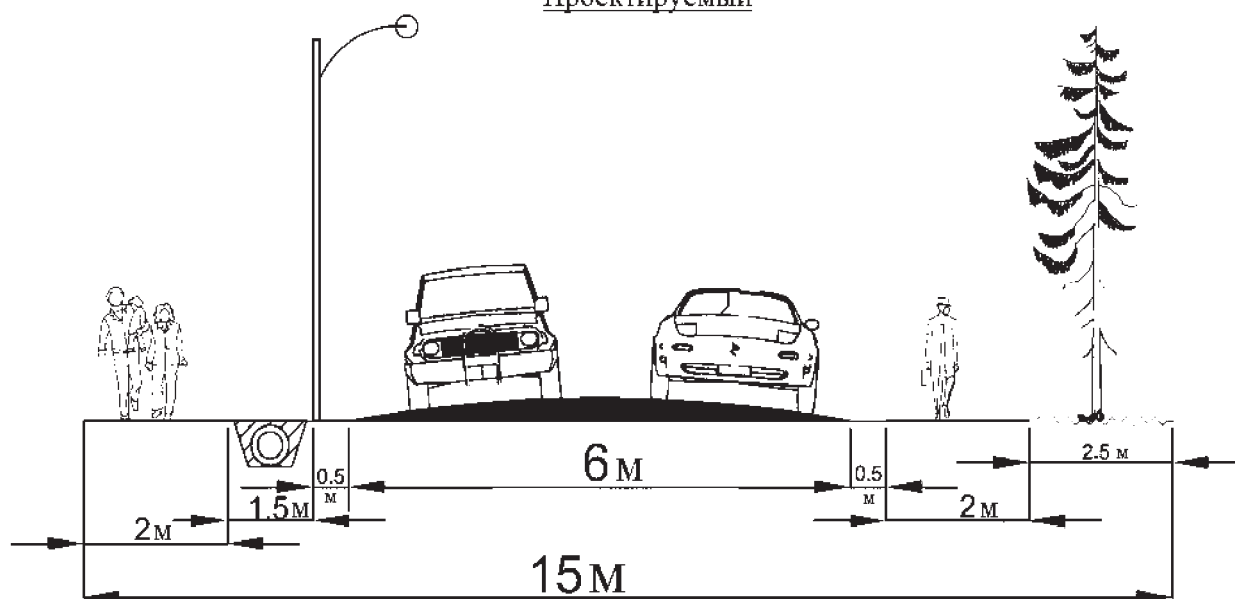
Поперечный профиль ул. Песчаная г. Елизово Проектируемый
