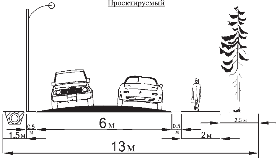
Поперечный профиль ул. Талалихина г. Елизово Проектируемый
