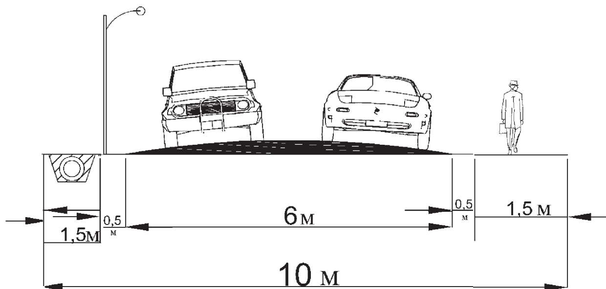
Поперечный профиль ул. Омская г. Елизово Проектируемый
