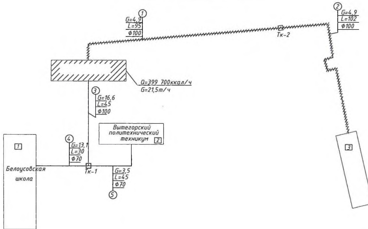
Схема тепловой сети котельной №17 в пос. Белоусово Анхимовского сельского поселения Вытегорского района
