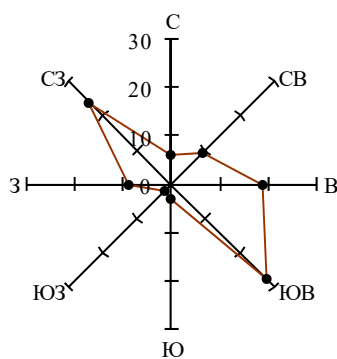
Роза ветров за холодный период по м/ст Иркутск, обсерватория
