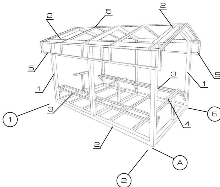
Рис. 45 – Конструктивная схема беседки для отдыха
