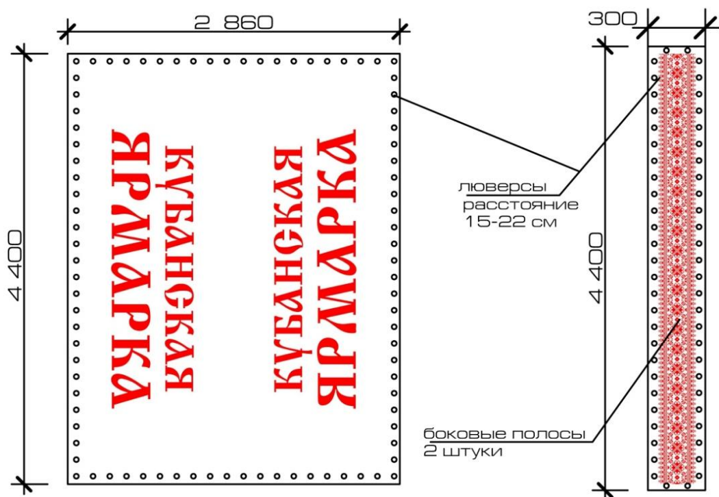
Рис. 51 – Схема кровельного баннера (натуральный размер)
