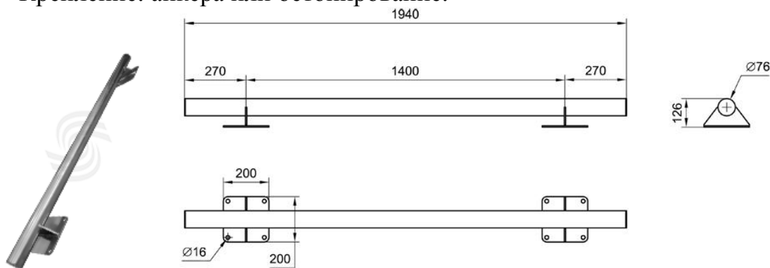
Рис. 17 – Пример колесоотбойника для парковки
