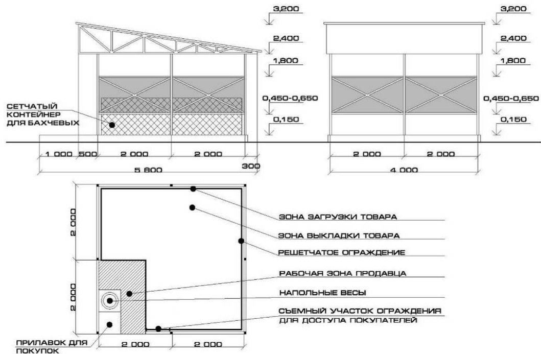
Рис. 27 – Вариант планировки торговой секции ярмарки
