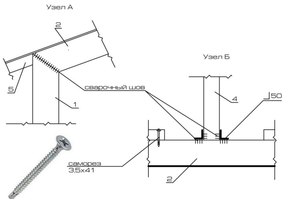
Рис. 50 – Узлы конструкции беседки для отдыха
