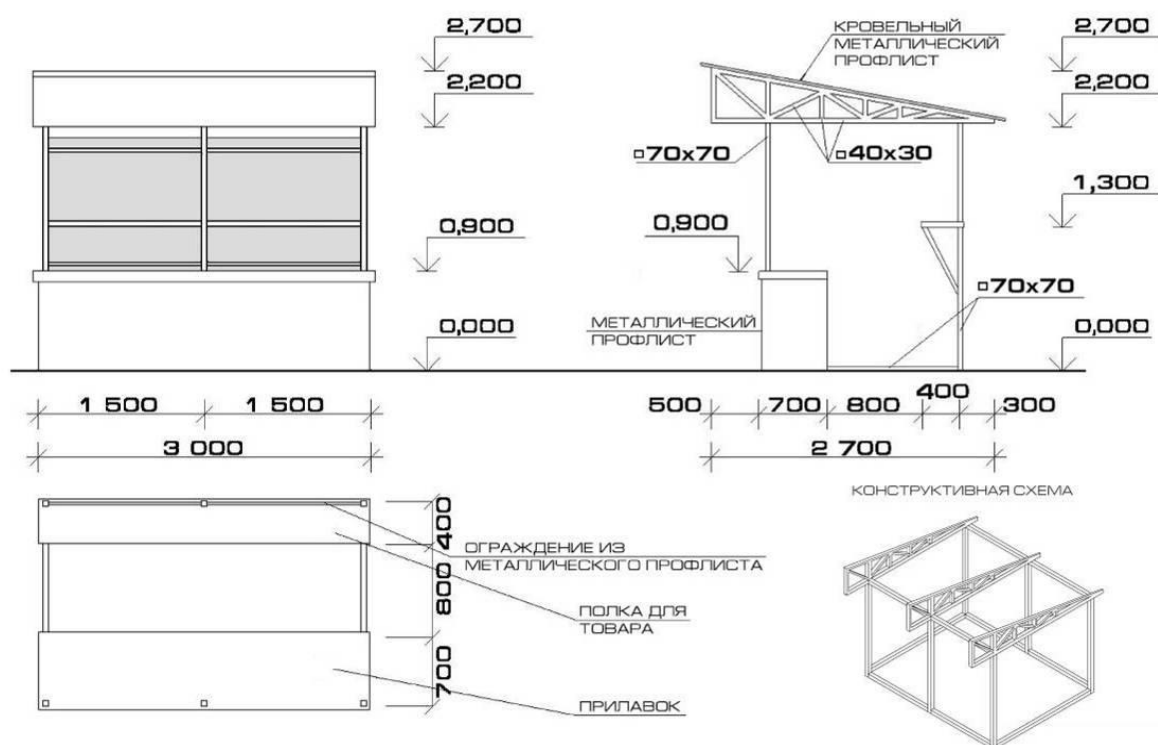
Рис. 62 – Планировка секции торговой секции «социального ряда»
