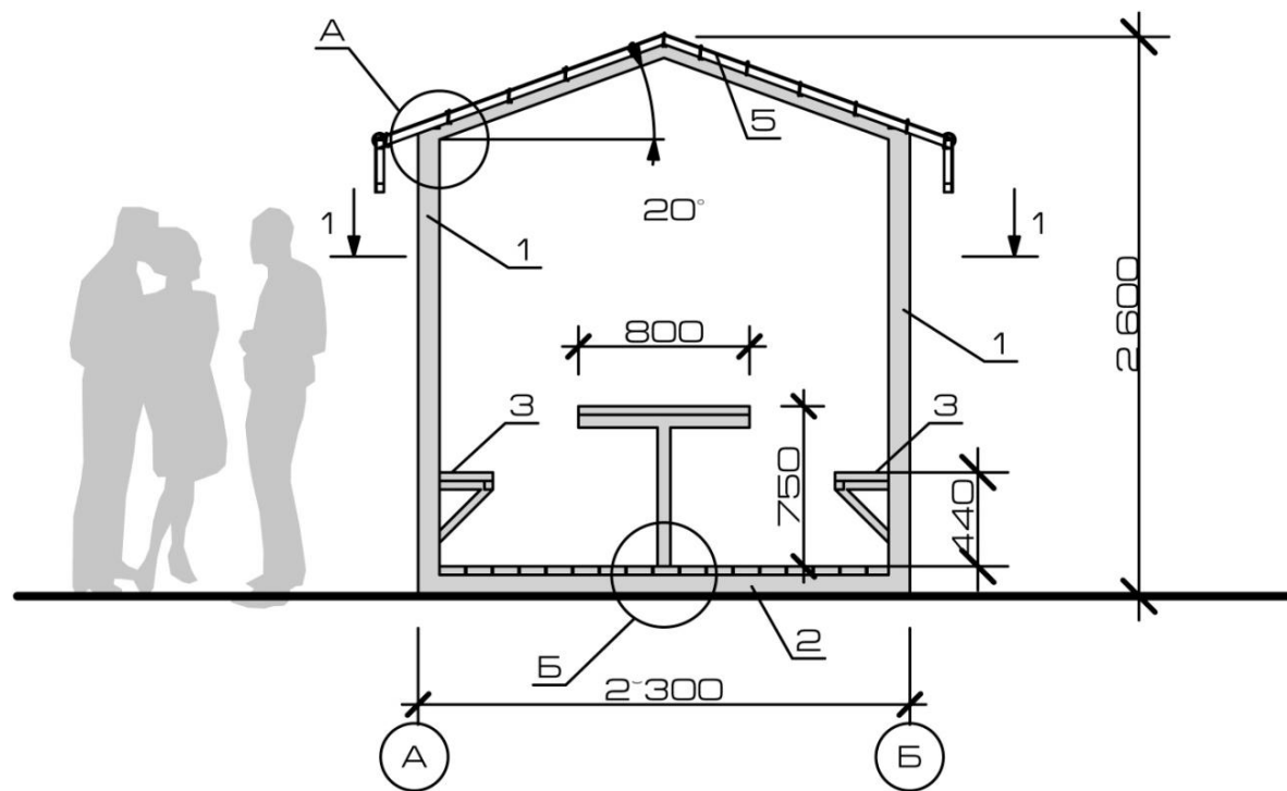
Рис. 48 – Боковой фасад
