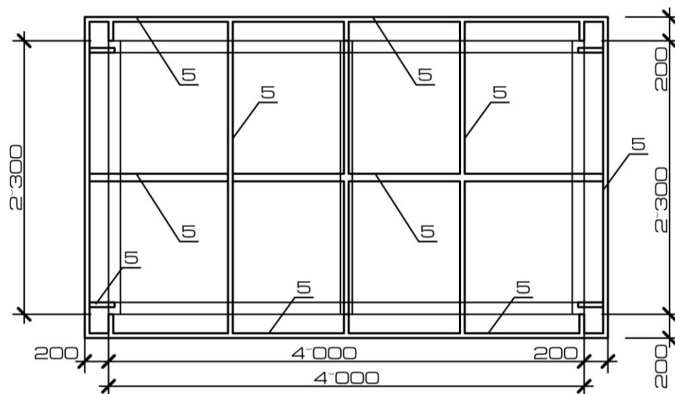
Рис. 46 – Схема конструктивных несущих элементов, мест для сидения и стола
