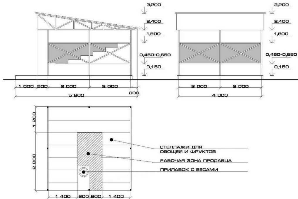
Рис. 26 – Вариант планировки торговой секции ярмарки
