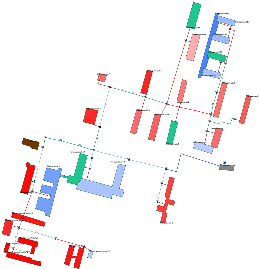
Рисунок 1.2 Схема тепловых сетей с отражением количества подведенного тепла по потребителям, типов прокладки и потерь напора по участкам сети зелёного цвета – получают расчетное количество теплоносителя; красного цвета – получают теплоносителя больше расчетного; синего цвета – получают теплоносителя меньше расчетного;
