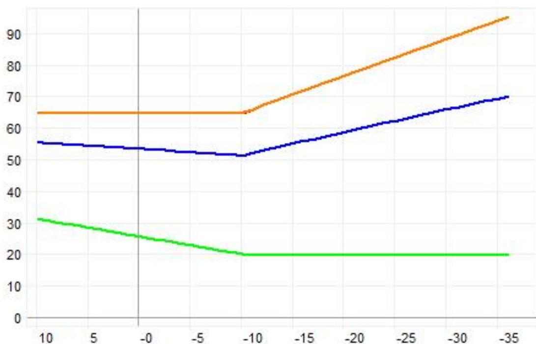
Рисунок 4.2 – Температурный график для потребителей после ЦТП 95/70 °С с полкой по подающему трубопроводу на 65°С
