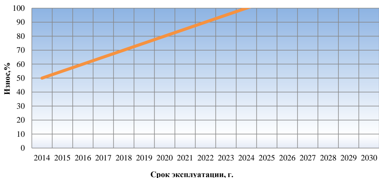
Рис. 7.1 – Зависимость износа тепловых сетей от срока эксплуатации
