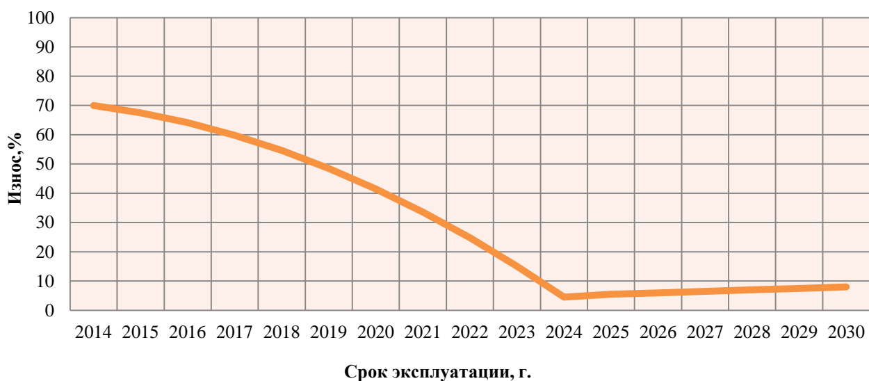
Рис. 7.2 - Зависимость износа тепловых сетей от срока эксплуатации
