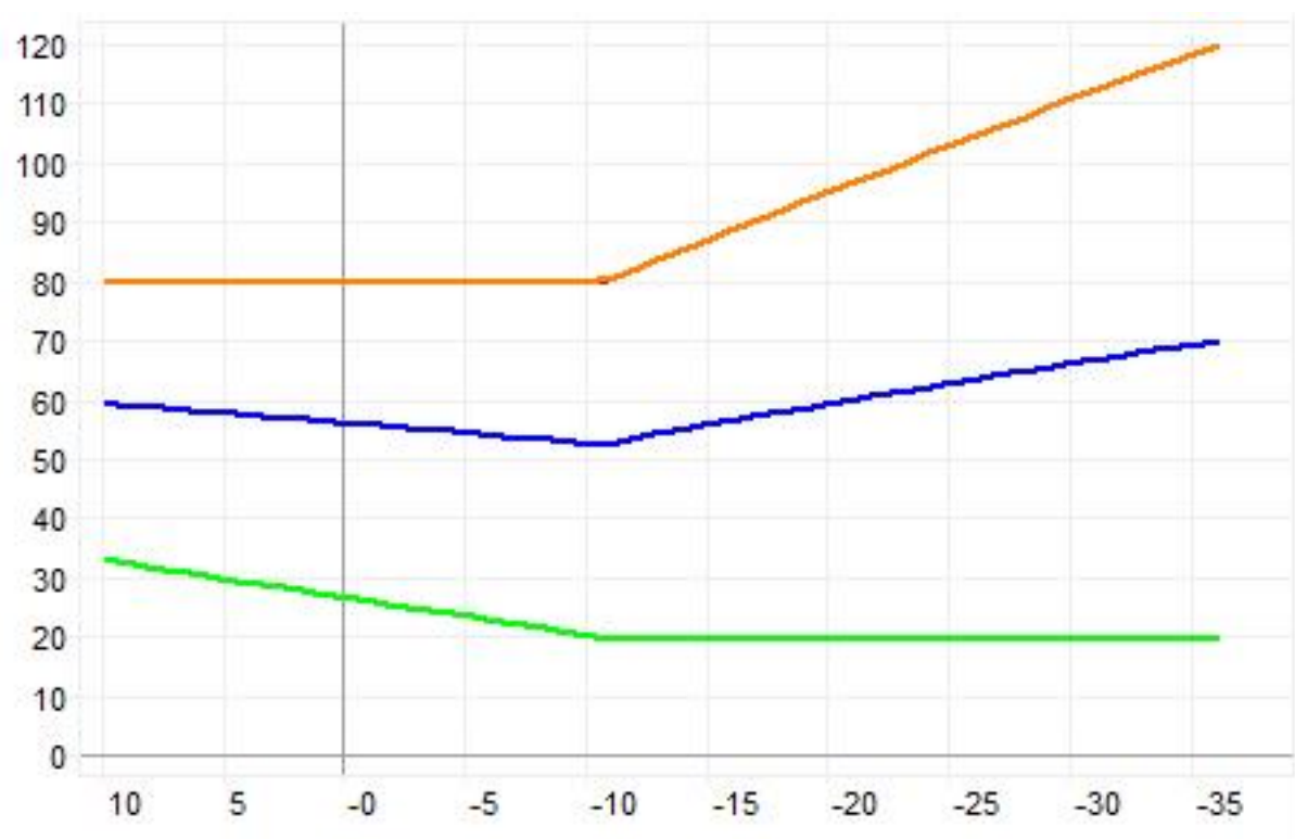
Рисунок 4.1 – Температурный график котельной 120/70 °С с полкой по подающему трубопроводу на 80°С
