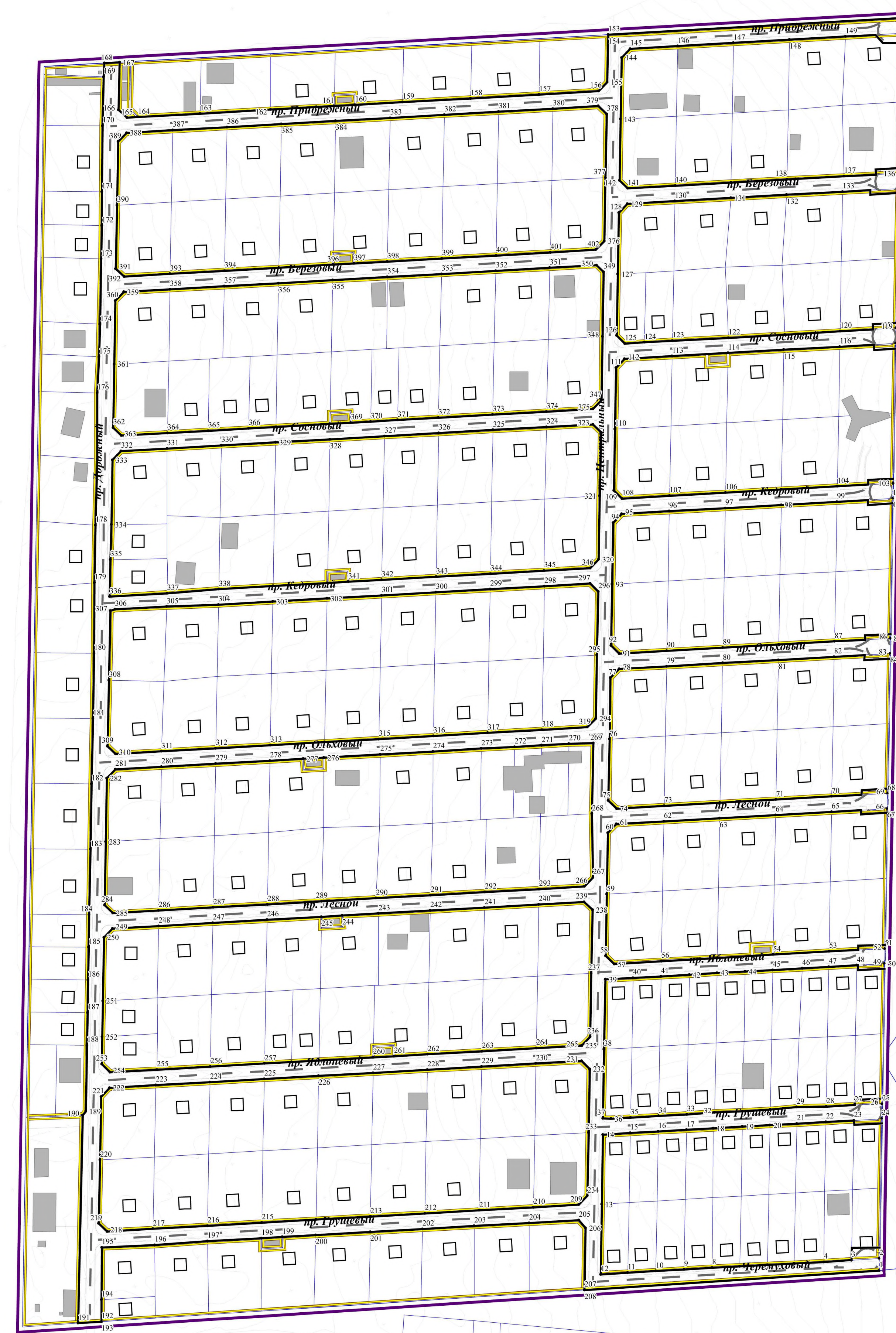
ПЛОЩАДКА №1 М 1:2 000
