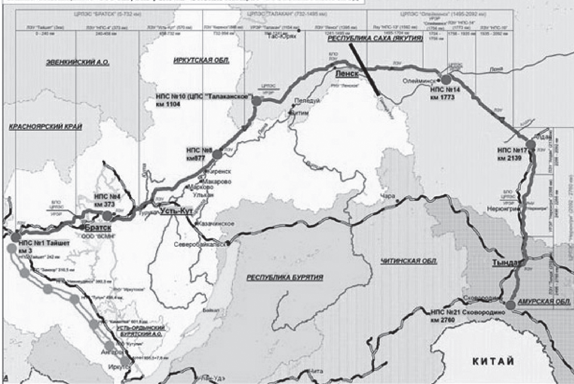
СХЕМА РАЗМЕЩЕНИЯ ООО МН, РНУ, СЛУЖБ ЭКСПЛУАТАЦИИ "ВОСТОКНЕФТЕПРОВОД"
