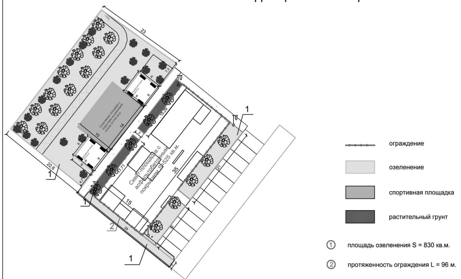
Схема устройства ограждений и озеленения общественной территории "Скейт-парк"
