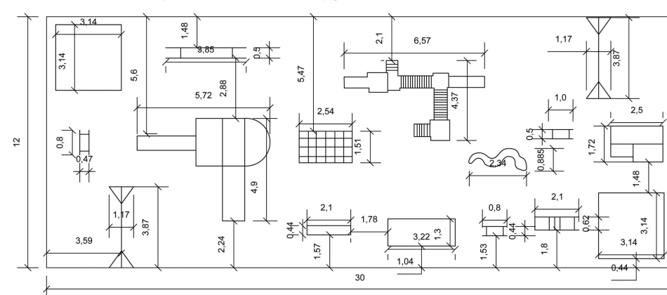
Схема размещения оборудования детской площадки
