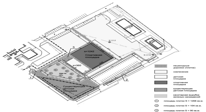
Схема устройства пешеходных дорожек общественной территории «ЗГГ микрорайон»
