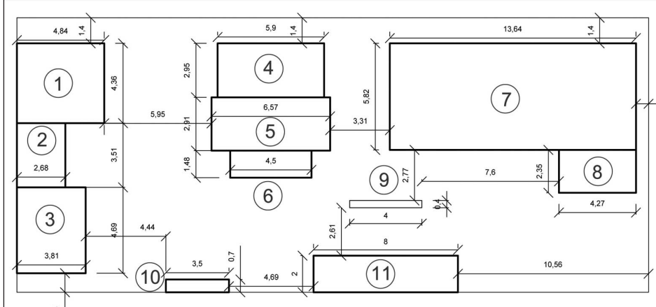
Схема размещения оборудования площадки для скейтборда
