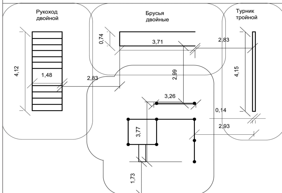
Элементы площадки для скейтборда
