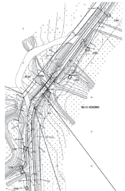
Чертеж межевания территории
