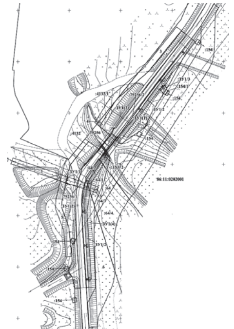
Чертеж границ земельных участков, используемых без предоставления земельных участков и установления сервитута
