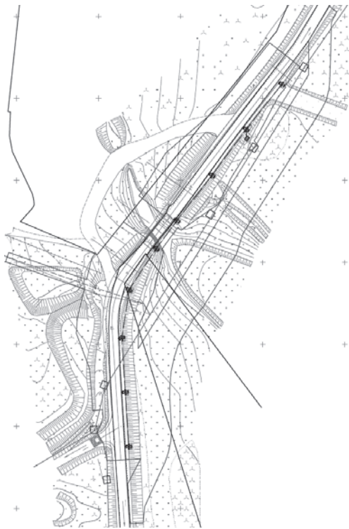
Схема размещения инженерных сетей и сооружений
