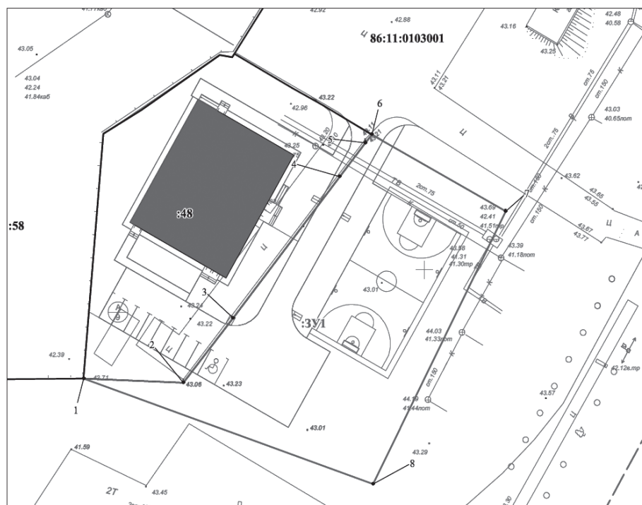
Чертеж образования земельного участка (2 этап)
