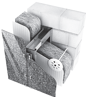
Рисунок 9.17. Отделка фасада керамогранитными плитами
