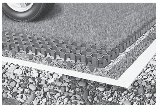
Рисунок 10.9. Устройство «Экопарковки»
