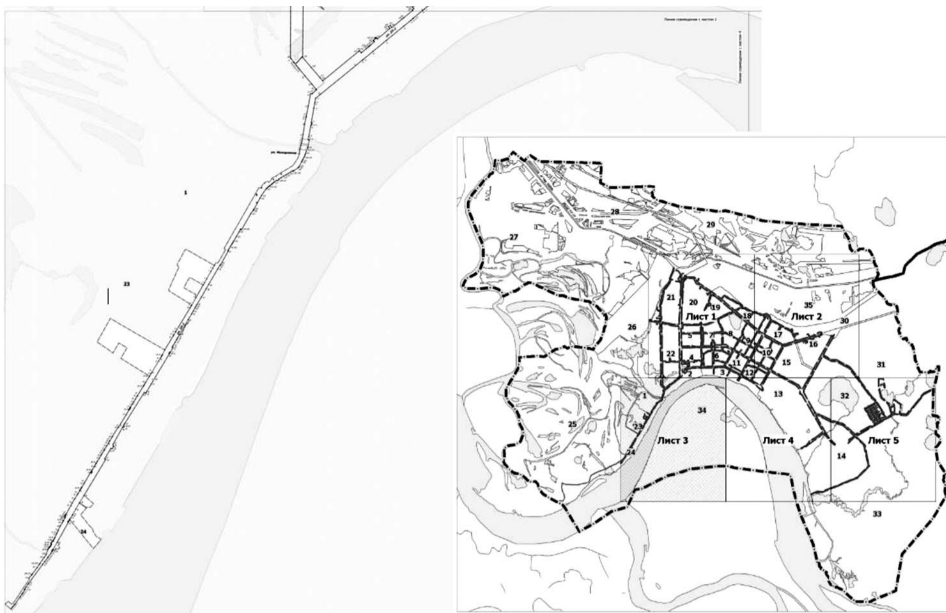
Чертеж межевания территории (II этап) (лист 2.4)
