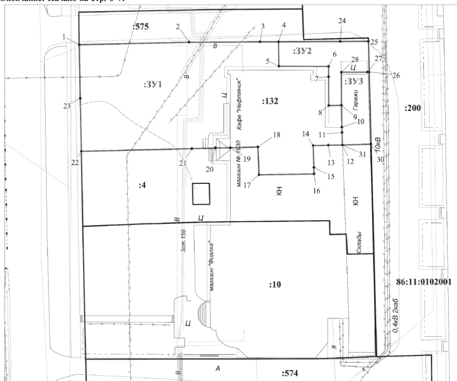
Чертеж образования земельных участков
