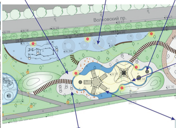
Сохранение всех здоровых деревьев, обрамляются покрытиями D1-1.2м
